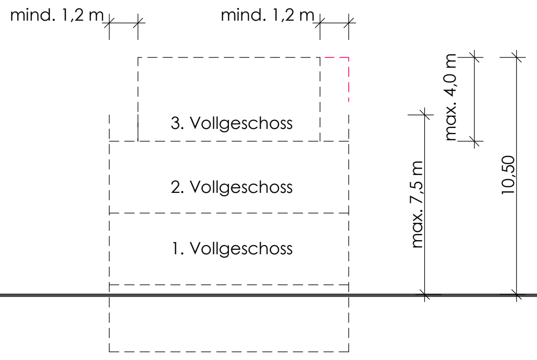
Variante: Attikageschoss
