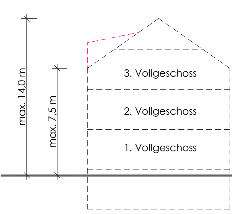
Variante: Satteldach
